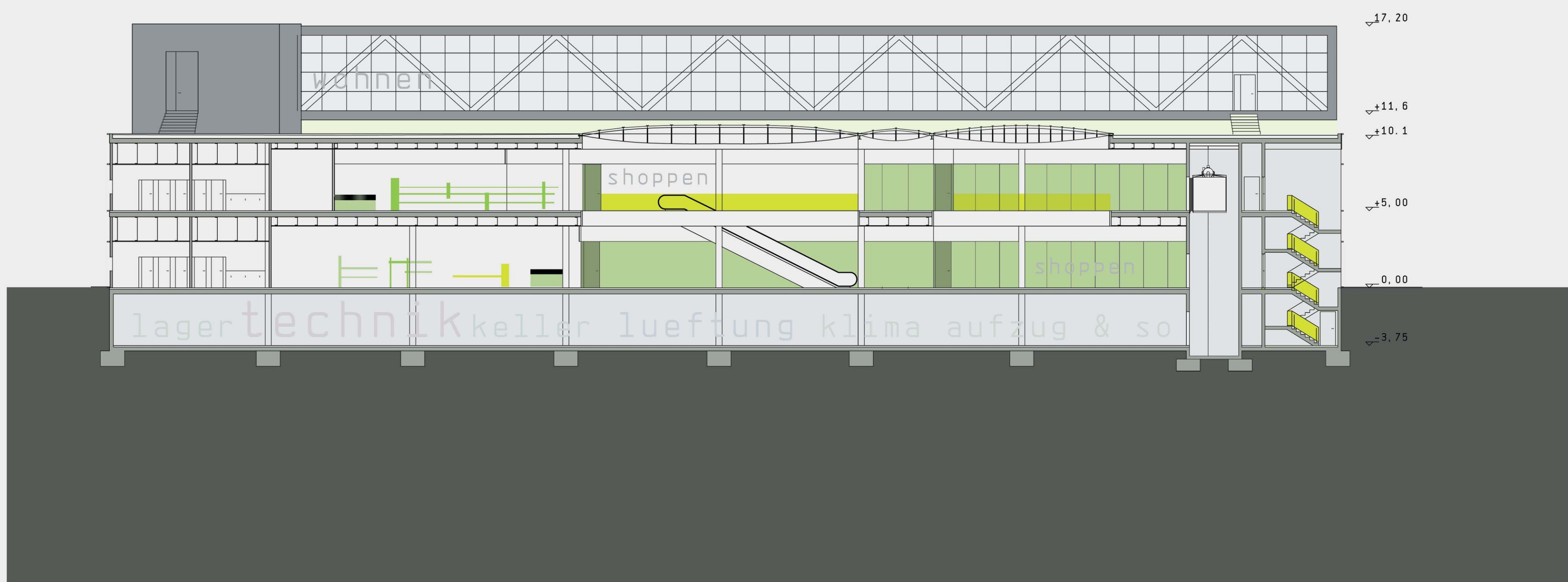
schnitt m 1:200
